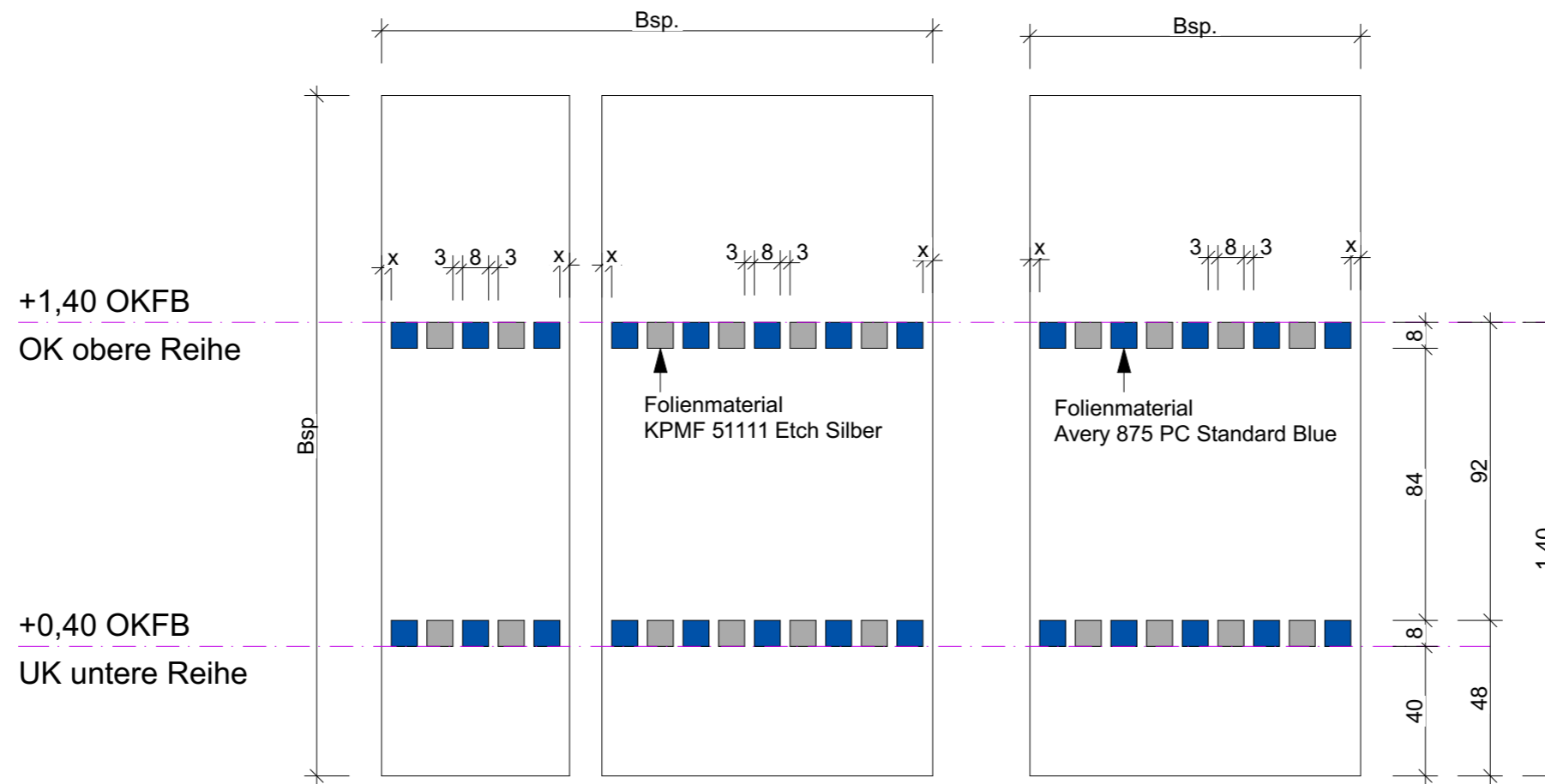
RS-Türen, zweiflügelig
